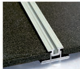
Eingelassene Bodenschiene mit Basisschiene
