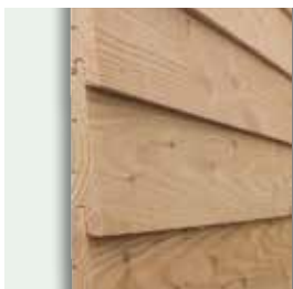
Fassadenprofil 28/15 x 142 mm, mit Nut und Feder, Sichtseite fein gesägt, technisch getrocknet
