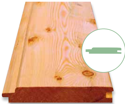
Rundkantenprofil im Schnitt: 19,5 x 96 mm mit Nut und Feder. Bsp. zeigt „Natur“ (Lärche).
