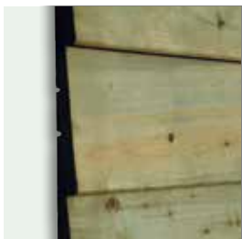
Fassadenprofil 28/19 x 146 mm, mit Nut und Feder, glatt gehobelt oder sägerau, trocken
