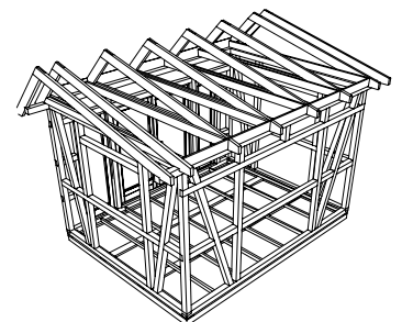
Grundgerüst 4 x 3 m
