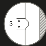
Prägung/Fräsung für Mala in Lavagrau in Millimetern
