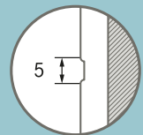
Prägung für Mala 14 und 18 in Millimetern
