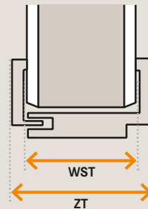
ZT: komplette Tiefe der Zarge WST: Wandstärke einschließlich Putz, Kacheln etc.
