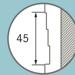
Fräsung für Sensa in Millimetern
