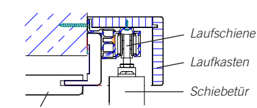
Montage mit Schiebetürfutter für Holztür
