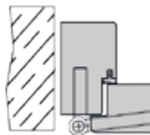
BLO - Blockrahmen Rahmenquerschnitt 65 x 75 mm
