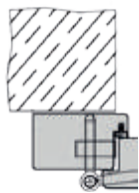
BLE - Blendrahmen Rahmenquerschnitt 75 x 44 mm
