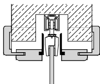
Schiebetür im Sturz für Glastür
