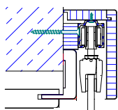
Montage mit Schiebetürfutter für Glastür
