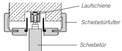
Schiebetür im Sturz für Holztür
