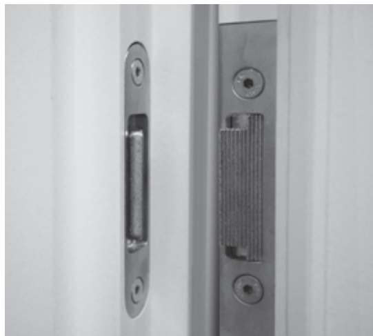
Bandseitensicherung Erschwert das Aushebeln einer Türe
