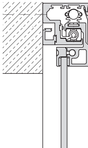
MOVE Montage Glastür ohne Futter mit Distanzprofil
