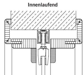
Glasschiebetür unter Sturz
