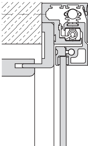
MOVE Montage Glastür mit Futter
