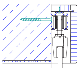
KLASSIK Wandmontage Glastür ohne Futter
