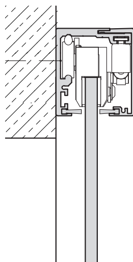
SLIM Wandmontage Glastür ohne Futter
