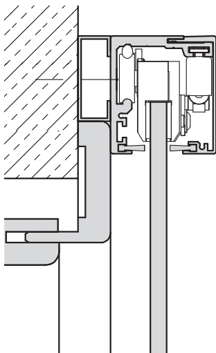
SLIM Wandmontage Glastür mit Futter und Distanzprofil
