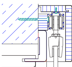
KLASSIK Wandmontage Glastür mit Futter
