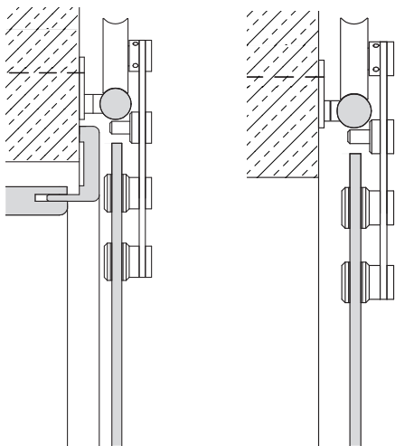
ART Montage Glastür mit Futter
