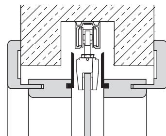
Glasschiebetür im Sturz
