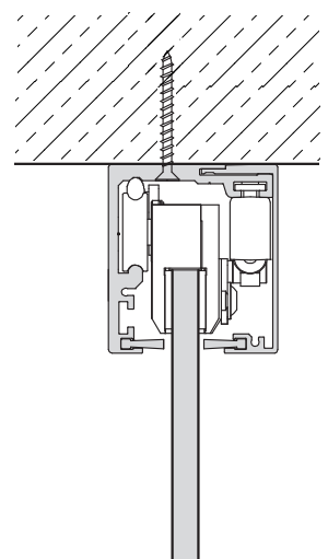
SLIM Deckenmontage Glastür ohne Futter
